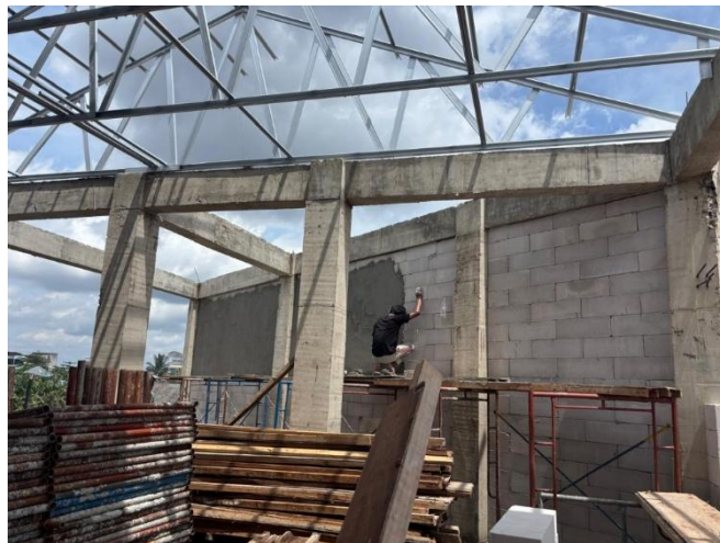
Gambar 7. Pekerjaan Plesteran Dinding
